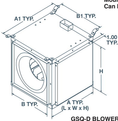
GSQ-D BLOWER
